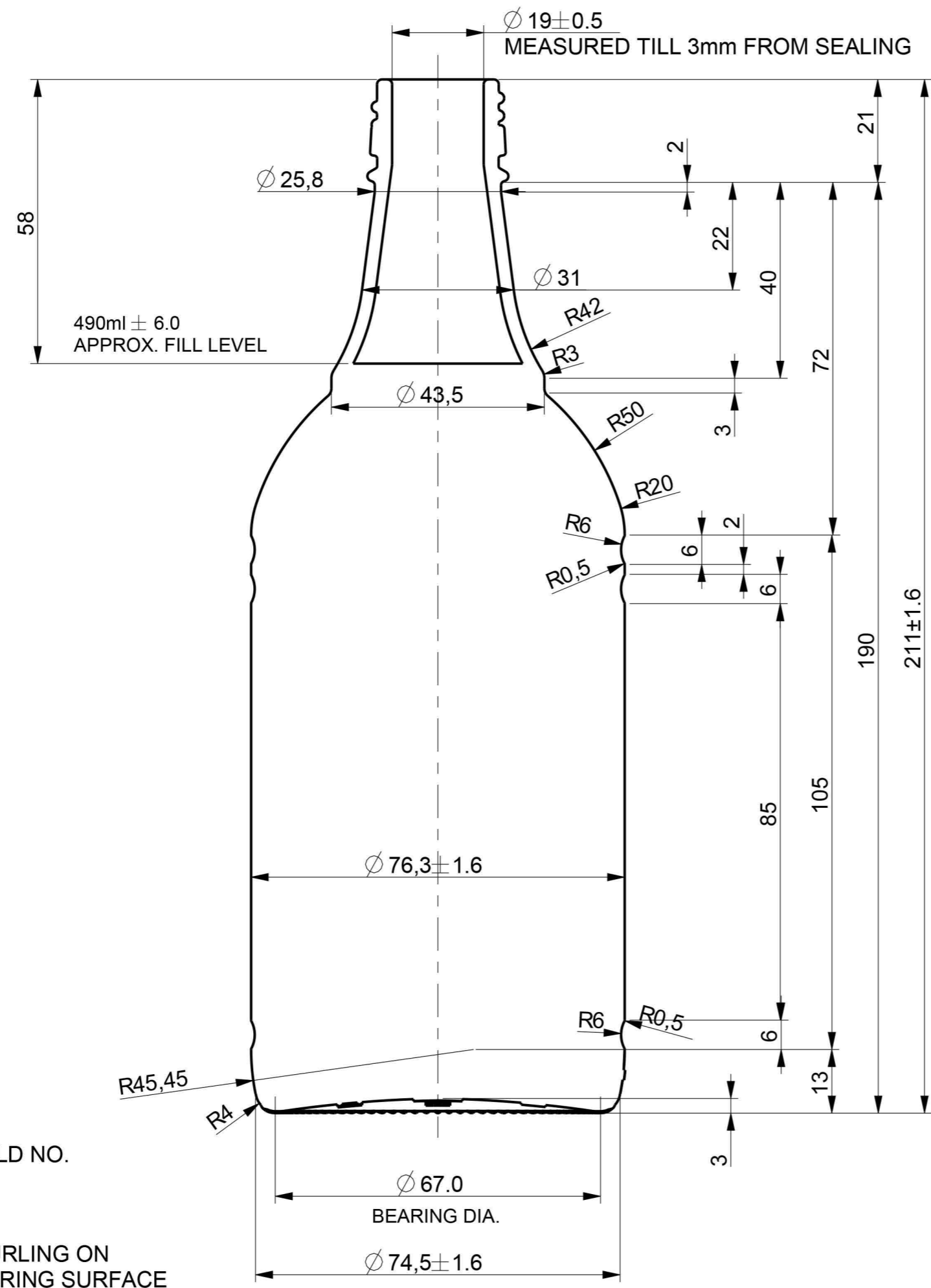
SECTION A-A
